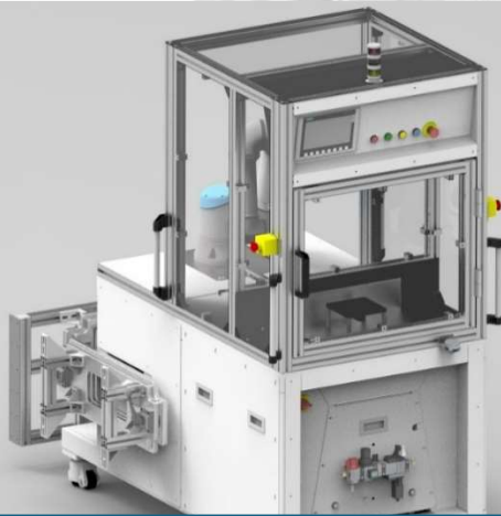
Robotkaros alapmodul
